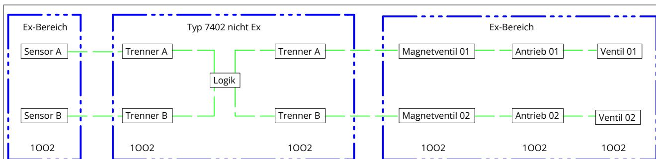
Bild 3: SIL 3 Verschaltungsschema zweikanalig
