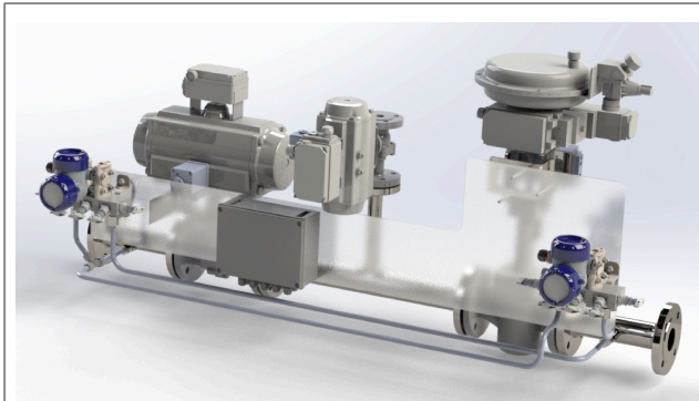
Bild 1: Zweikanalige Rückströmsicherung Typ 7305
